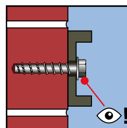
4. Erop letten dat kop goed aansluit → Klaar.
