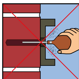
2. Boormeel hoeft niet te worden verwijderd!
