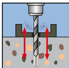
2. Nettoyer le trou
