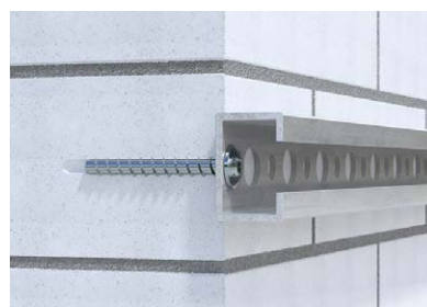
Fixation de rails de montage
