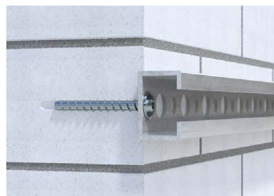
Montage van montagerails
