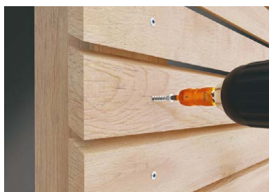
Vissage de façades
