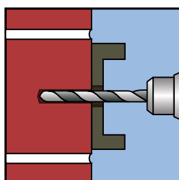
1. Boorgat maken (klopboor)
