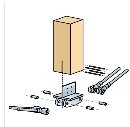
Onderspannen ligger
