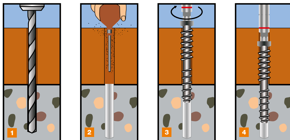
1. Boren
