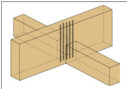
Dwarsaansluitingen
