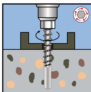
3. Inschroeven
