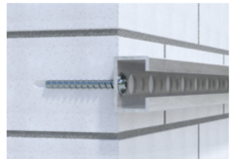
Montage van montagerails
