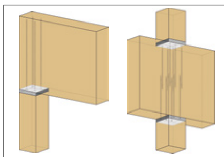
Draagvlakversterking
