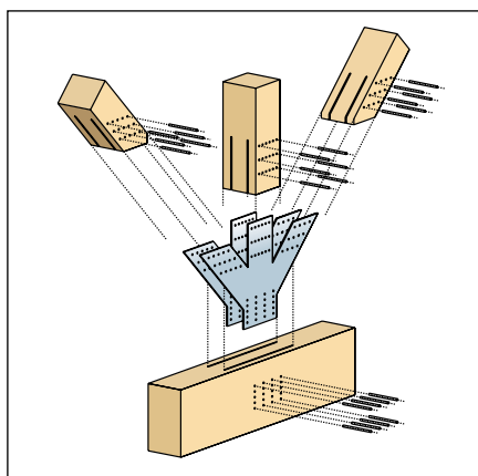
Vakwerk-Knooppunt
