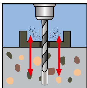
2. Boorgat schoonmaken
