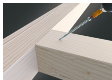
Hoofdhulpligger verbinding
