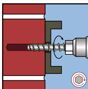
3. Inschroeven (schroefboormachine)
