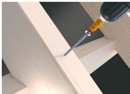
Spantbevestiging
