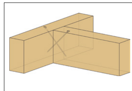
Hoofd-/hulppliggers
