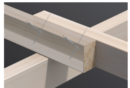
Koppelde kruisverbinding
