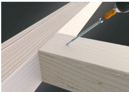
Hoofdhulpligger verbinding
